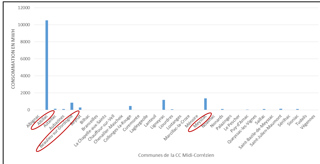
Consommations électrique liées à l'industrie sur la Communauté de communes Midi Corrèzien (Source: AREC, 2017)
