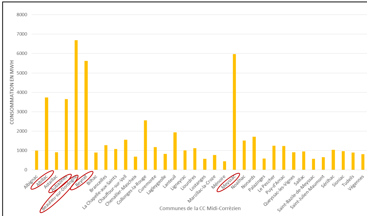
Consommations électrique liées au secteur résidentiel sur la Communauté de communes Midi Corrèzien (Source : AREC, 2017)
