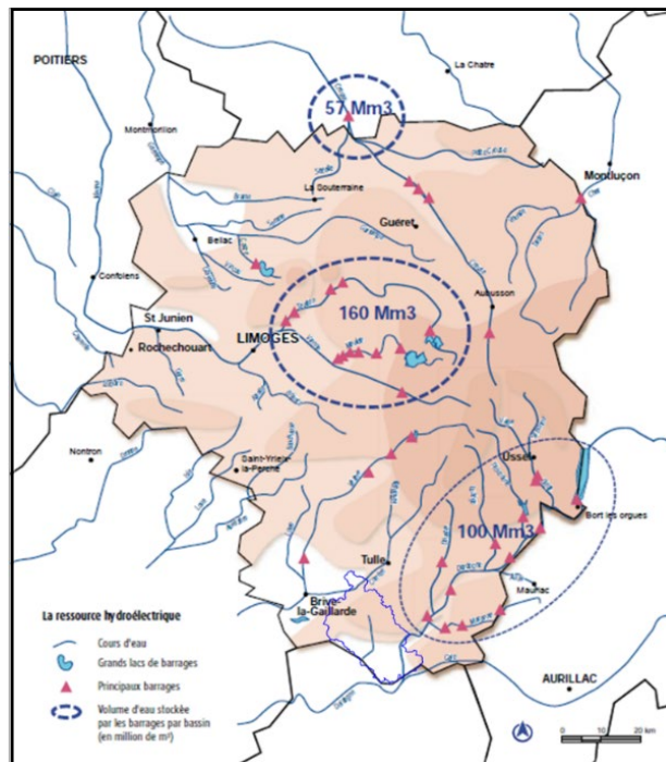
Les ressources hydroélectriques sur l'ancienne région Limousin (Source: DREAL Limousin, Agence de l'eau)
