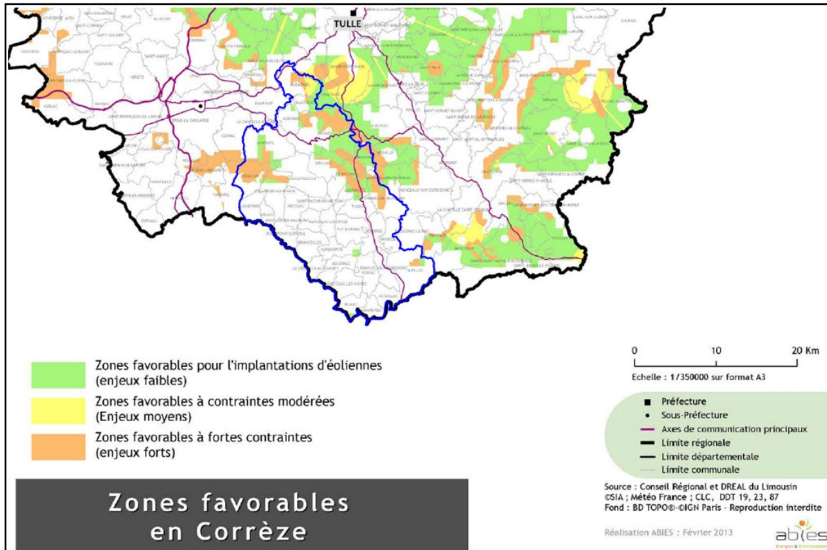
Extrait carte représentant les zones favorables à l'implantation d'éoliennes sur le département de la Corrèze (Source : SRE Limousin 2013)
