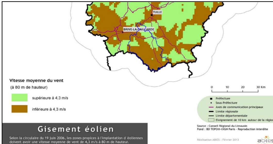
Extrait carte représentant le gisement éolien sur l'ancienne région Limousin (Source: SRE Limousin 2013)
