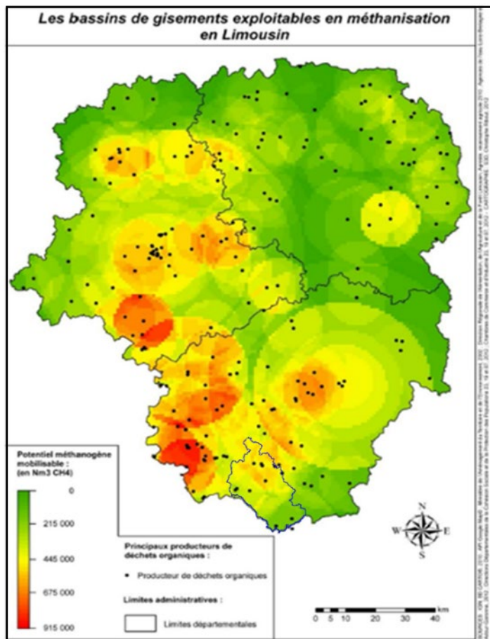
Gisements exploitables en méthanisation dans le Limousin (Source : S3d étude méthanisation Limousin)
